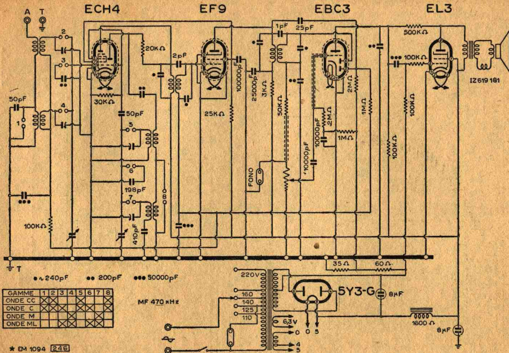
Lo schema elettrico del Phonola 585
